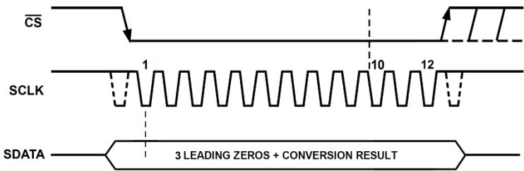
时序图
