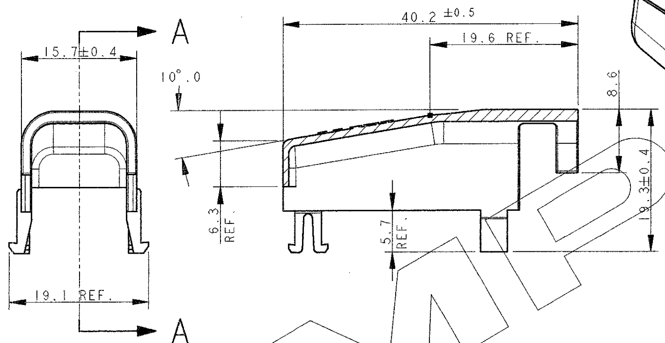
SECTION A-A ( SEZIONE A-A )
