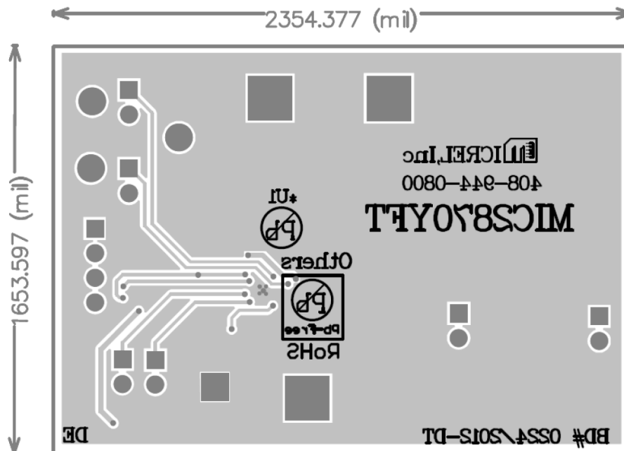
Bottom Layer
