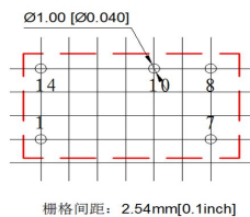
推荐 PCB 图
