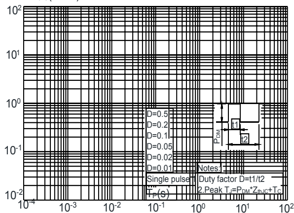
Z_{th_{J-C}} (^{\circ}C/W)
