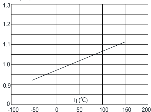
V_{BR(DSS)}
