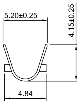
SEC:B-B
