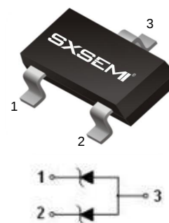
SOT-23
