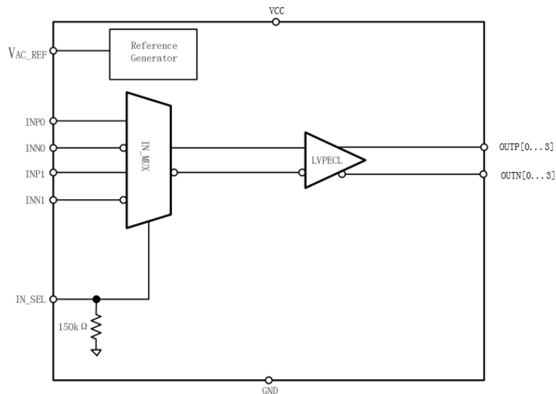
图1 功能框图
