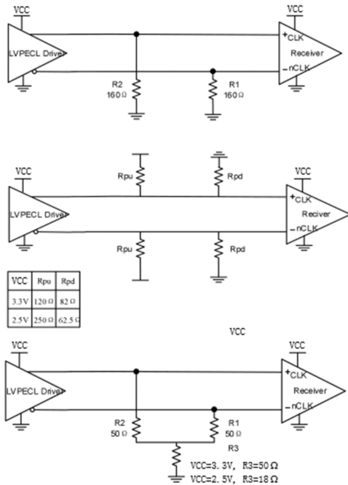
图11 LVPECL 驱动器
