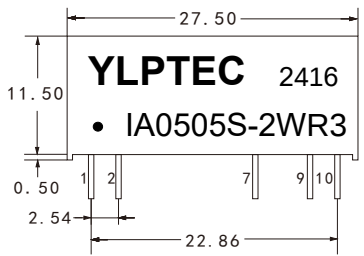
1) 外观尺寸
