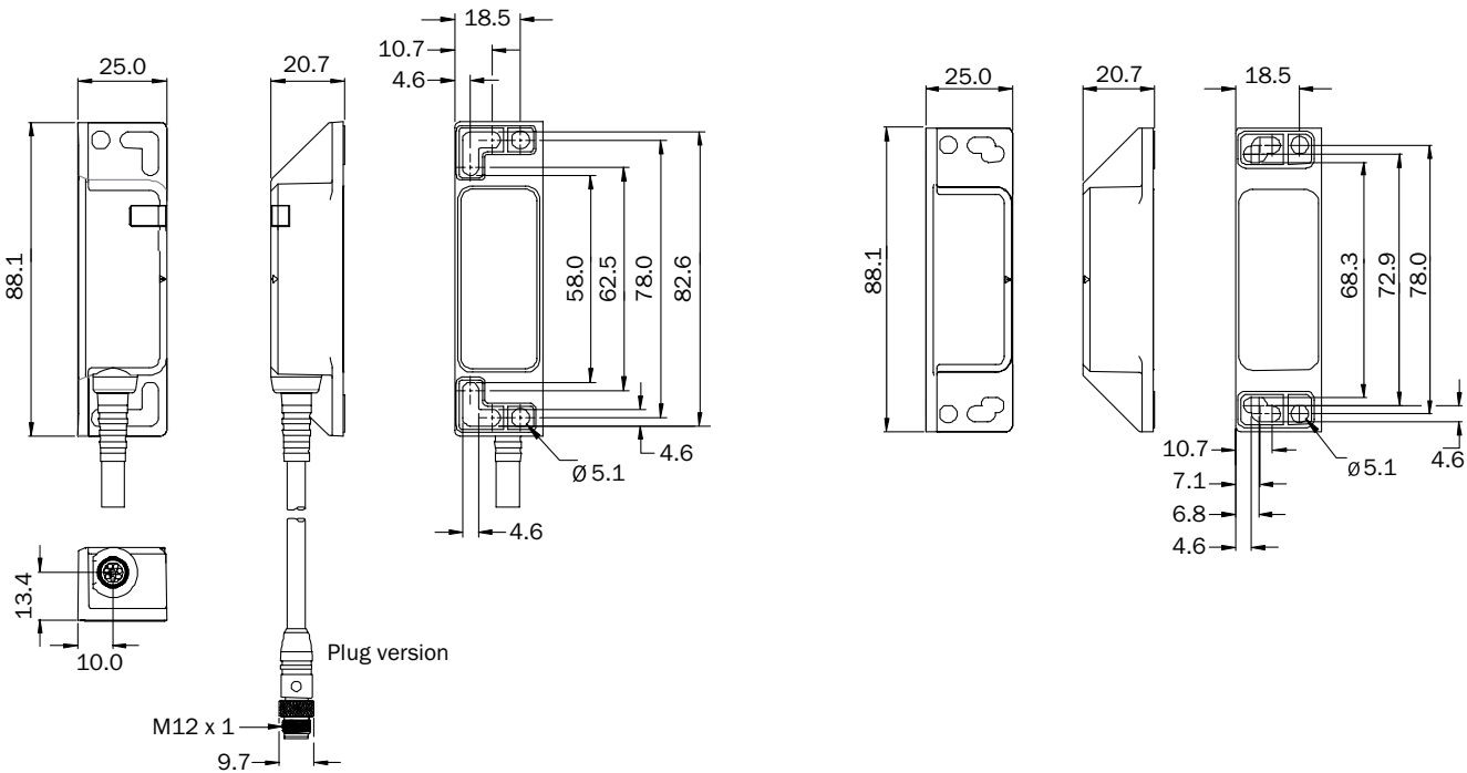
尺寸图 (尺寸单位: mm)
