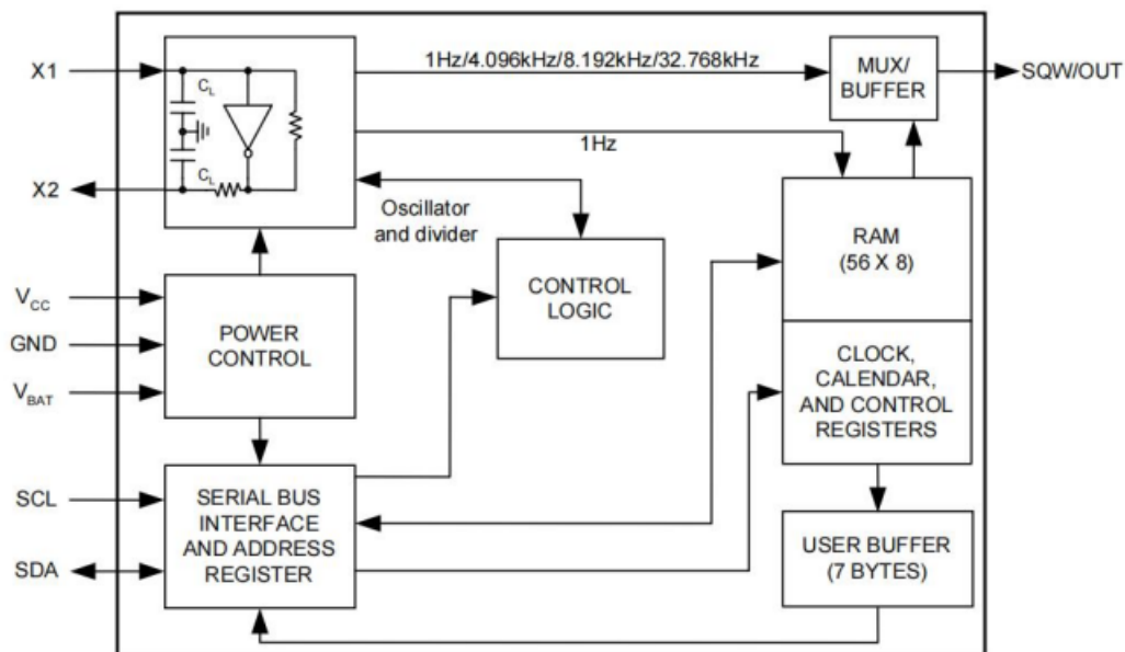
图1 内部功能框图
