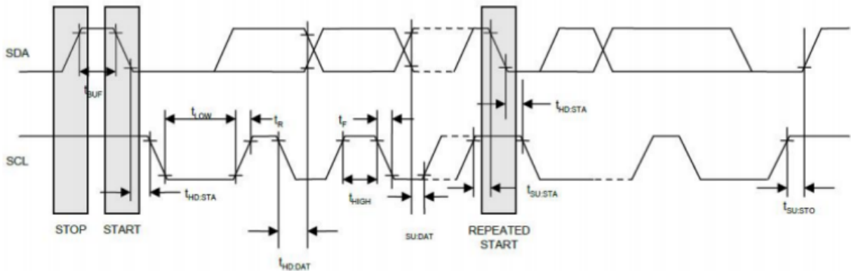
图 3 时序图
