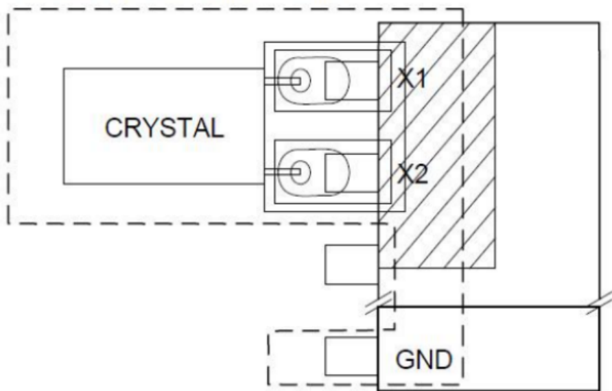
图4 晶振印刷电路板布局
