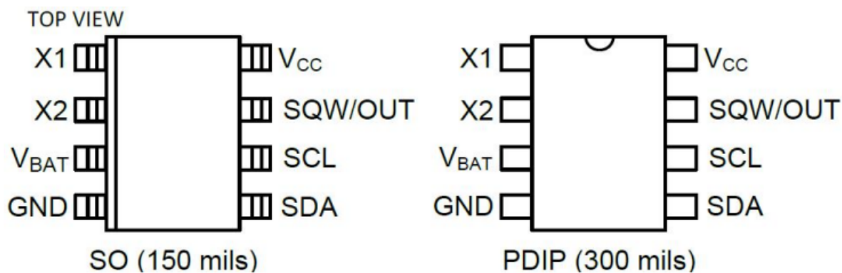
图 2 管脚排列图
