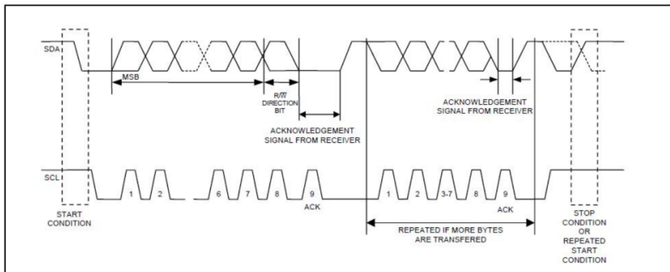
图 5 IC 串行总线上的数据传输
