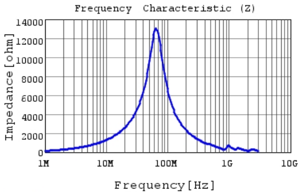
LQW43FT220M0H |Z|
