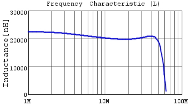
LQW43FT220M0H L
