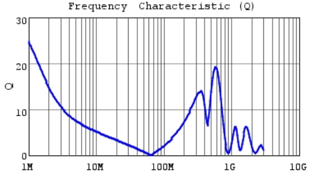
LQW43FT220M0H Q
