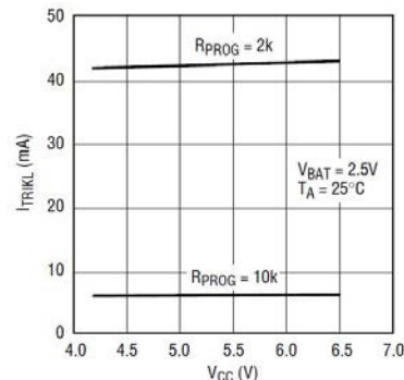
充电电流 vs 电源电压
