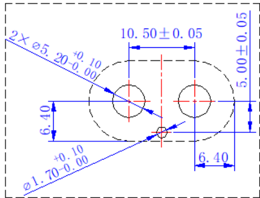
互配尺寸
