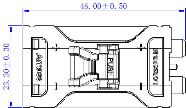
互配尺寸
