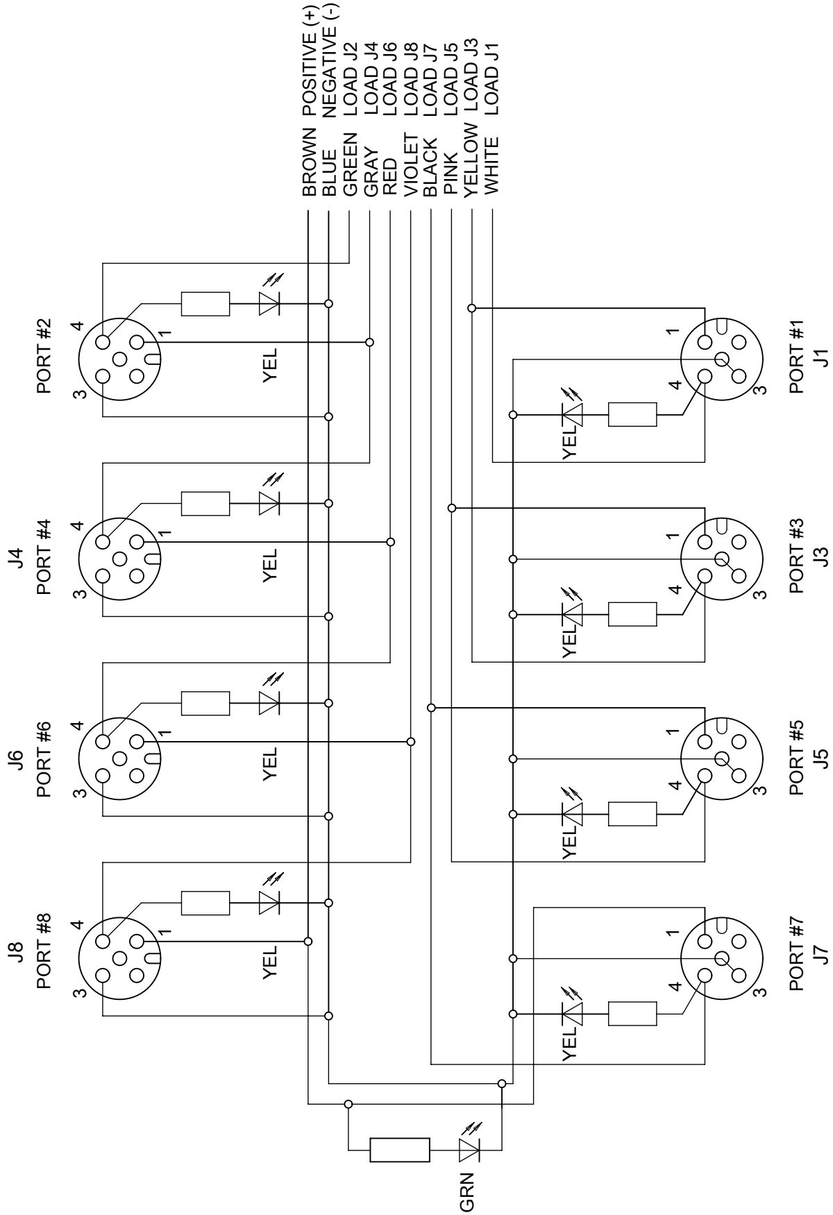
WIRING SCHEMATIC
