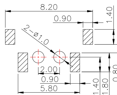
PCB.焊接图
