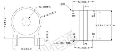
主视图
