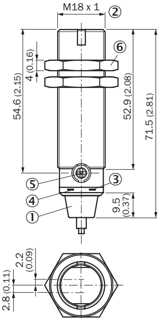
尺寸图 (尺寸单位: mm) GRTE18, GRL18, GRSE18, 金属, 电缆, 轴向
