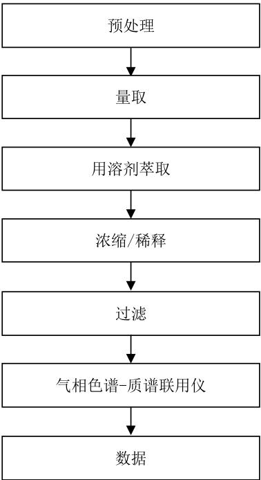
PBB/PBDE/Phthalates 检测流程图
