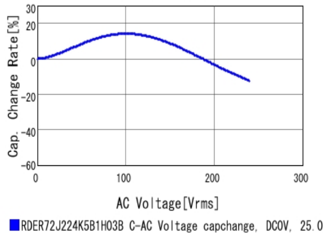
交流电压特性
