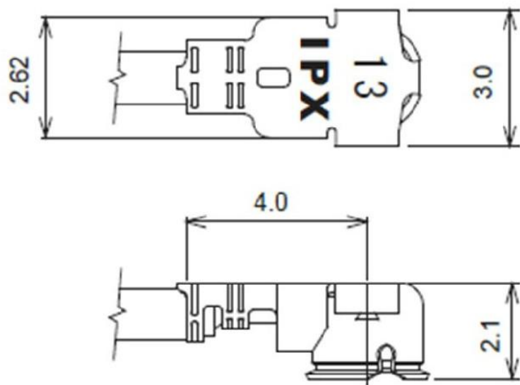
图 8 天线扣规格图
