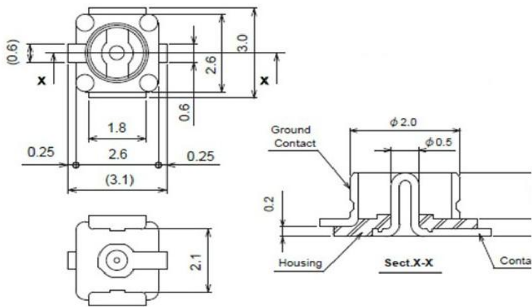
图 7 天线座规格图
