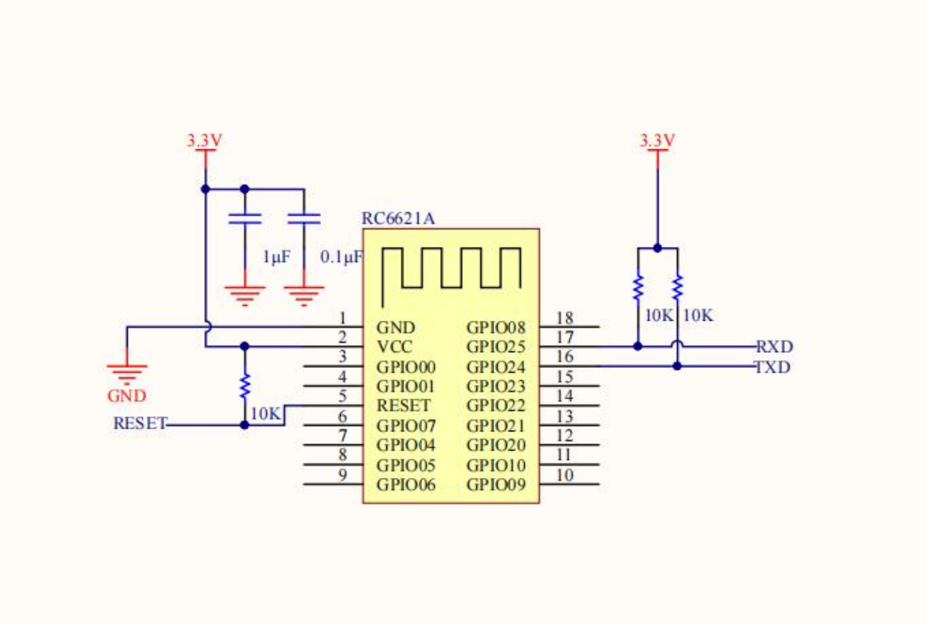
图 6 模块外围推荐按电路
