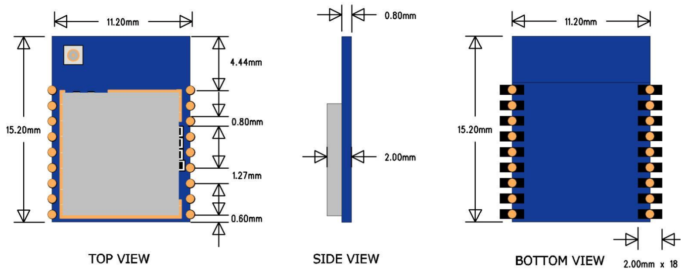
图 4 模块尺寸图
