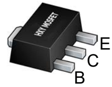
SOT-89 (TO-243AA)
