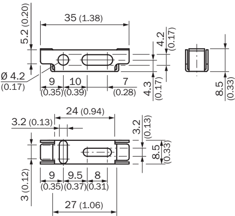
尺寸图 (尺寸单位: mm)
