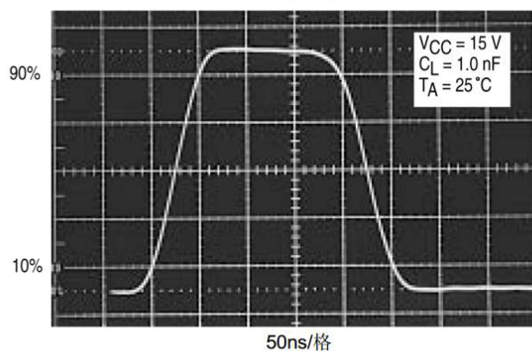
图 12. 输出波形
