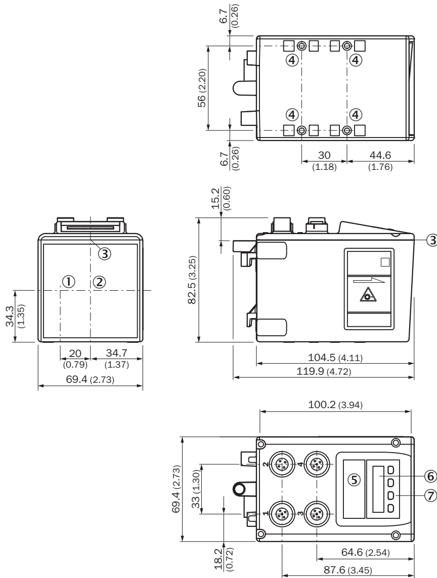
尺寸图
