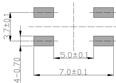
P.C.B 板焊接图
