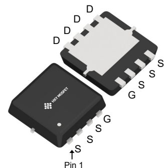
DFN3X3-8L (PowerDI333-8)
