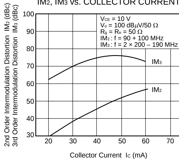
IM 2 , IM 3 vs. COLLECTOR CURRENT
