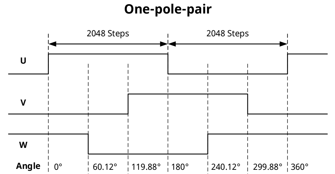
图 9：1 对极 UVW 波形图
