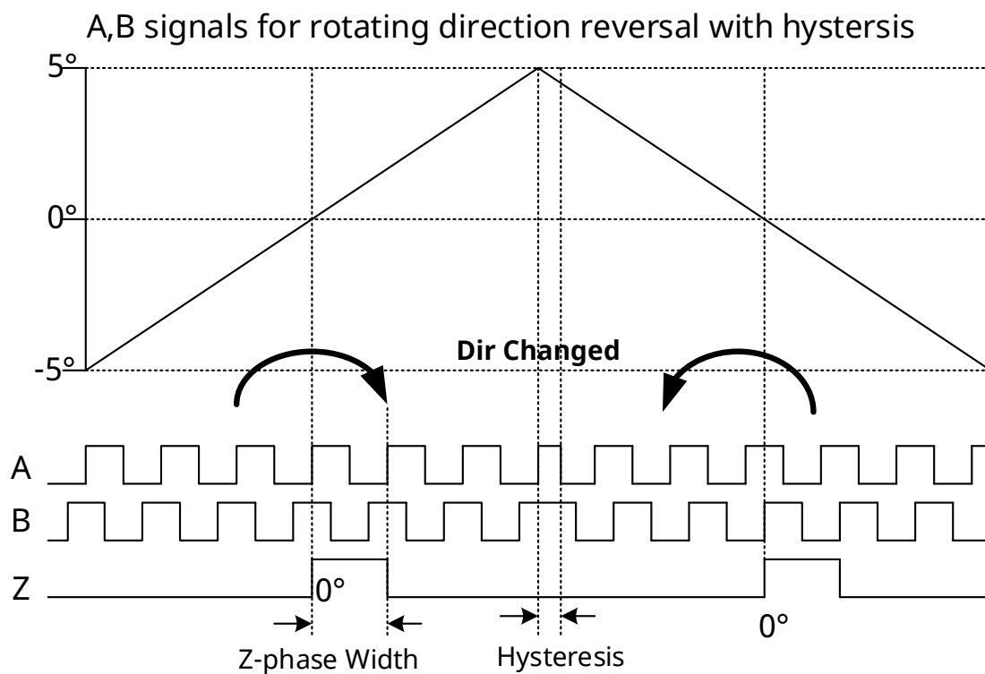
图 8：脉冲波形图
