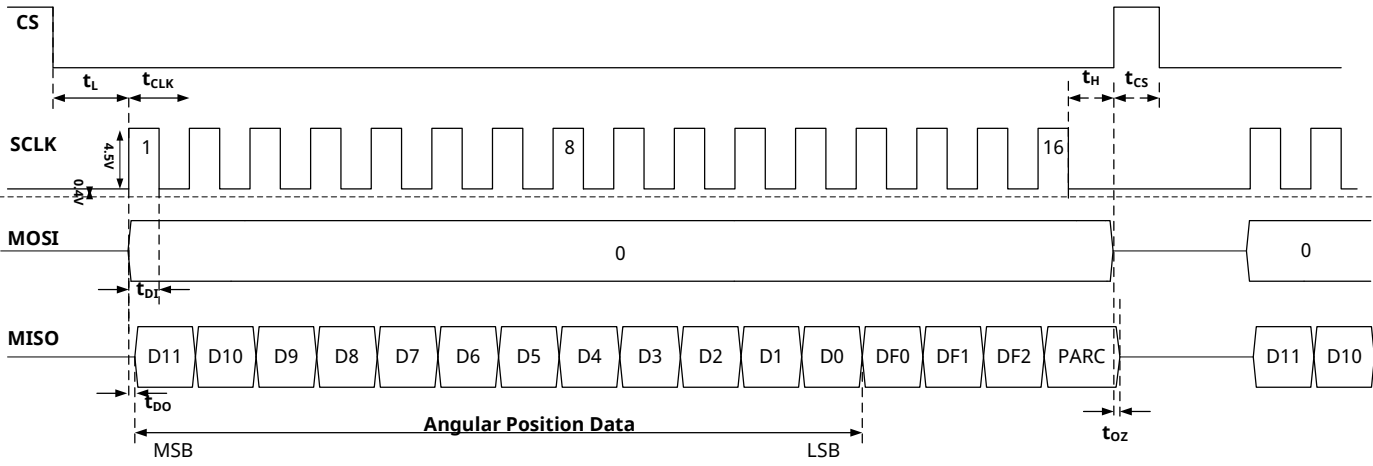
图 7：SPI 时序图
