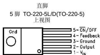
LM2576T-XX/NOPB 或 LM2576HVT-XX/NOPB
