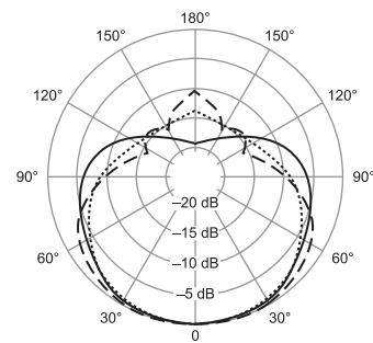
— 2000 Hz ..... 4000 Hz --- 8000 Hz TYPICAL POLAR PATTERNS COURBE DE DIRECTIVITE TYPQUES - TYPISCHE POLARCHARAKTERISTIK PATRONES DE CAPTACION POLAR TIPICOS - TIPICI DIAGRAMMI POLARI 指向特性
