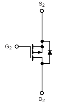
P-Channel MOSFET
