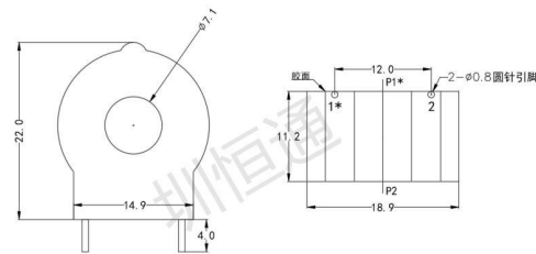
主视图
