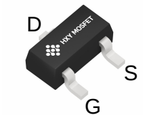
SOT-23 (SuperSOT-6)
