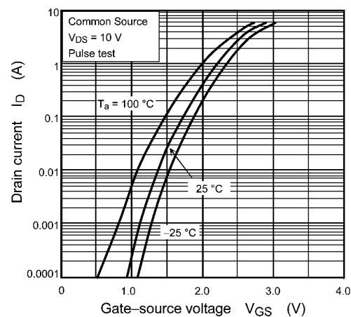
Fig. 7.2 I_D - V_{GS}
