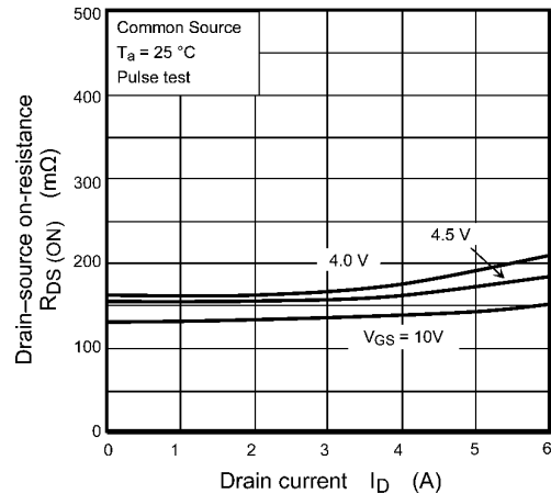
Fig. 7.4 R_{DS(ON)} - I_D
