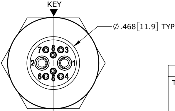
WIRING END W7A82-8SG-P-300 SHOWN
