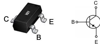
SOT-23
