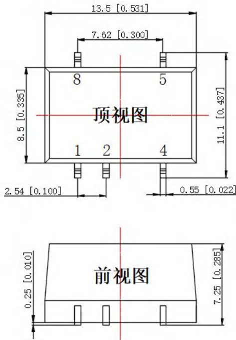
外观尺寸图
