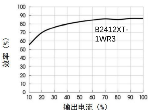
效率 VS 输出负载电网图（Vin=24V）
