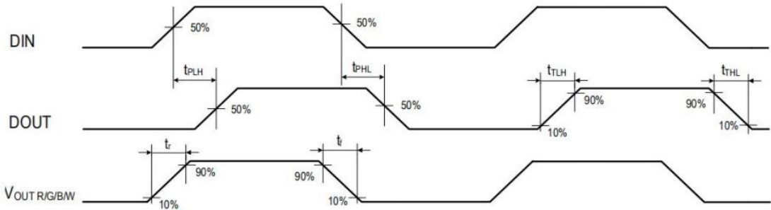
动态参数测试示意图
