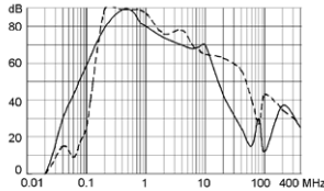
36A (FMBC-0940-3610L)
