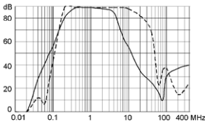
50A (FMBC-0938-5010L)
