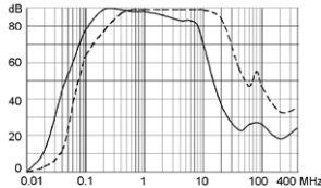
36A (FMBC-0940-3610L)
