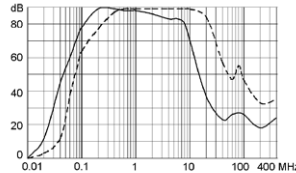
50A (FMBC-0938-5010)
