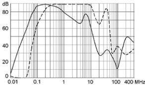
25A (FMBC-0932-2510L)
