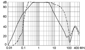
50A (FMBC-0938-5010)
