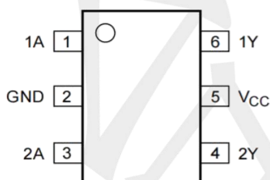
SOT363
