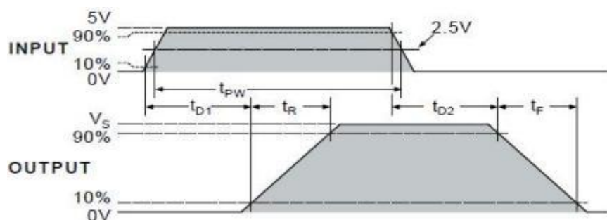
输入输出（B通道同相）波形图
