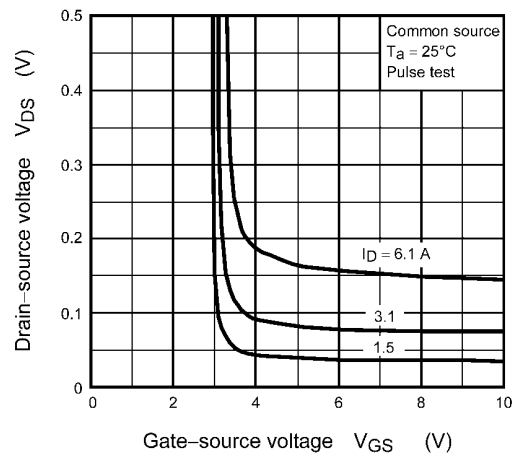
Fig. 8.2.4 V_{DS} - V_{GS}
