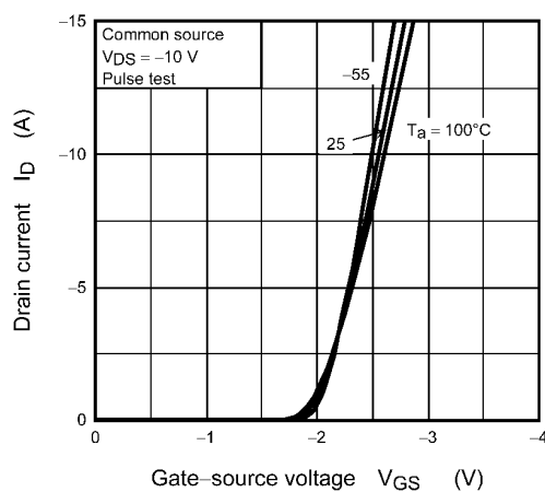
Fig. 8.1.3 I_D - V_{GS}
