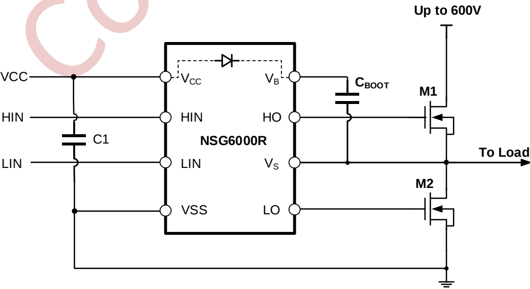
图 10-2 NSG6000R 典型应用电路图
