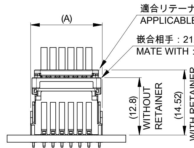
4 ISLタイプ嵌合図 MATED CONNECTOR OF ISL TYPE
