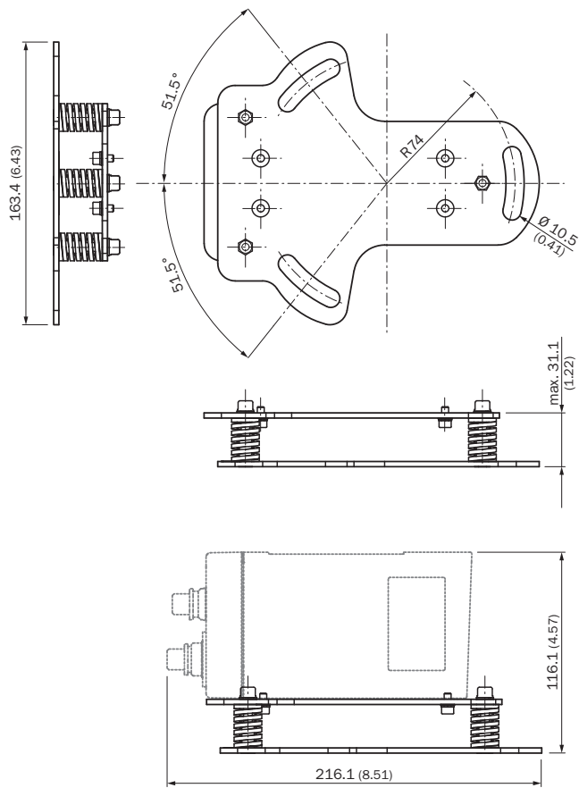
尺寸图 (尺寸单位: mm)
