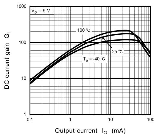
Fig. 7.4 G_I - I_O
