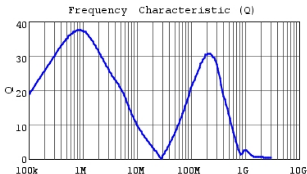
LQH3NPZ220MJR Q
