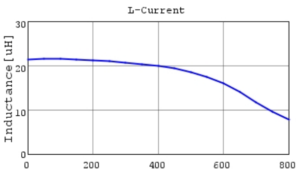
LQH3NPZ220MJR L-Current 20degC
