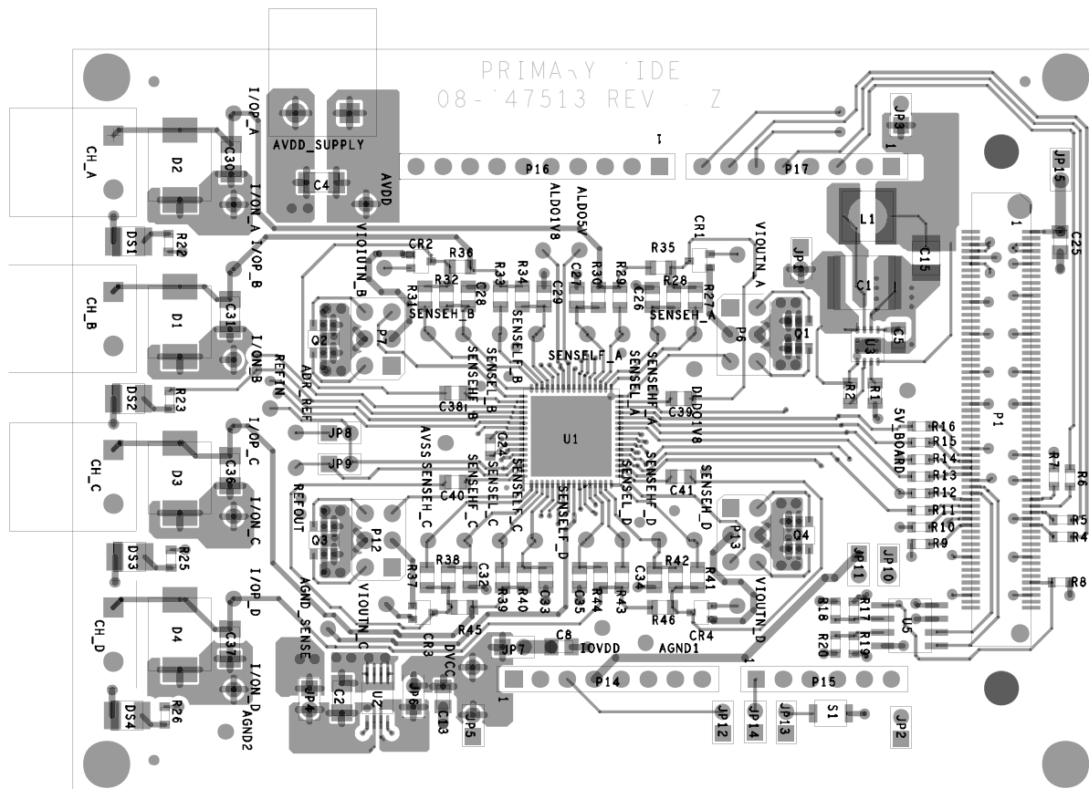
Figure 14. Layer 1, Top Layer
