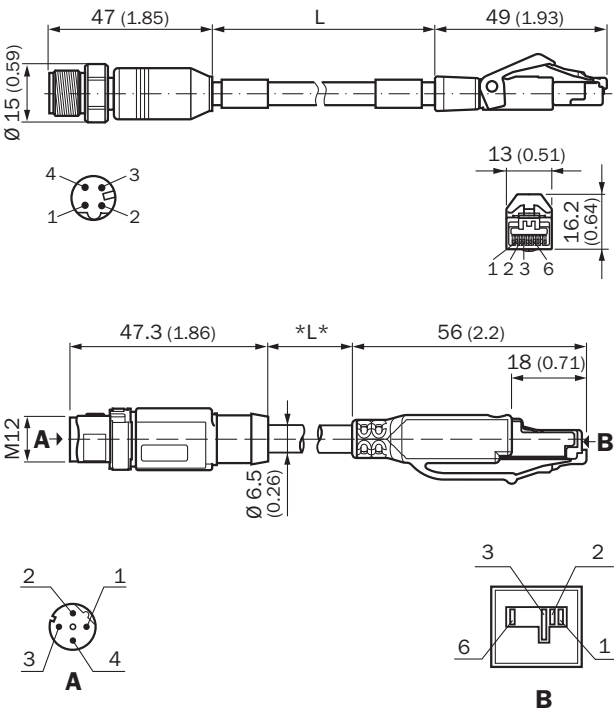
尺寸图 (尺寸单位: mm)
